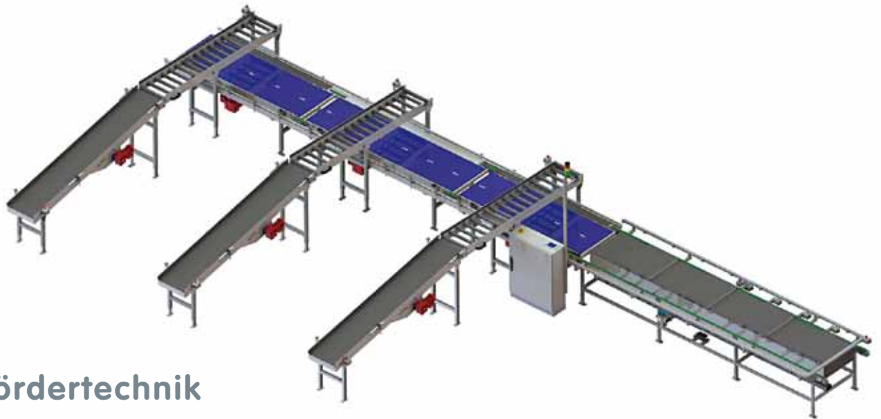
WA Förderanlage - Briefsortierung
